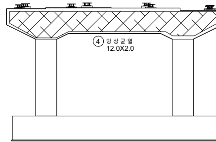
배면
